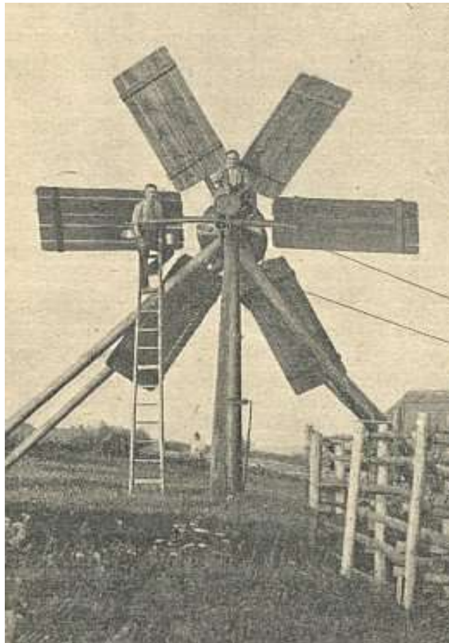
Dřevěná větrná turbína v Dolní Pestřici
